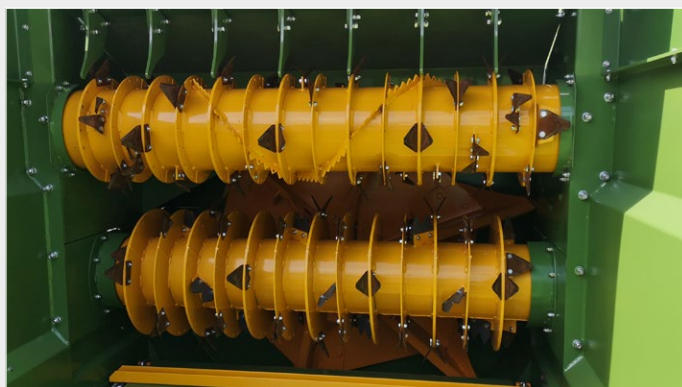
Rozdružovací válce umístěné nad sebou
